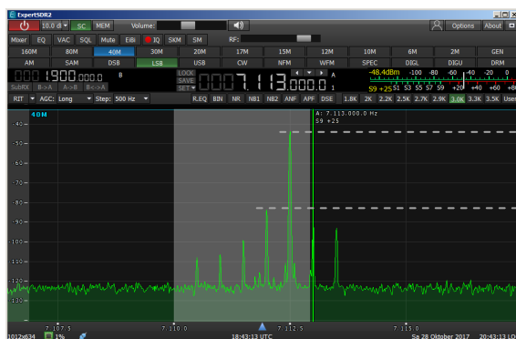
Bild 7: NF-Klirrfaktor, 1%
